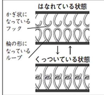
面ファスナーの仕組み
